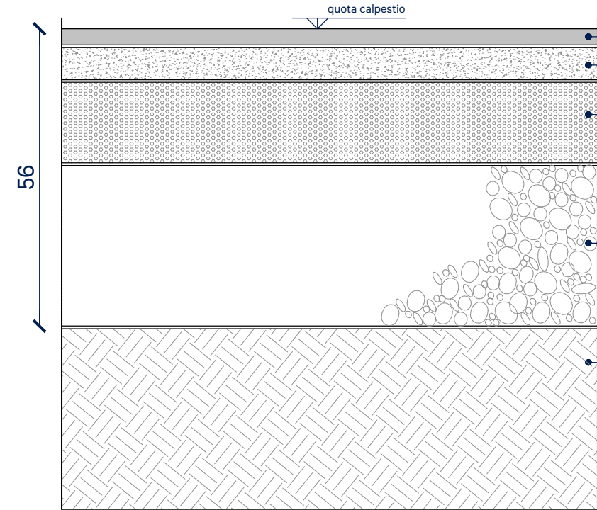
C01 - Pavimentazione in calcestruzzo drenante scala 1:10
