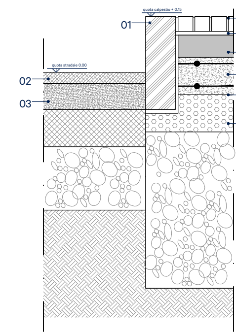
C04 - Dettaglio cordolo in granito scala 1:10
