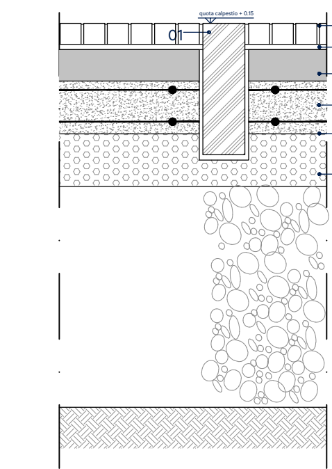
C04 - Dettaglio bindero a raso scala 1:10
