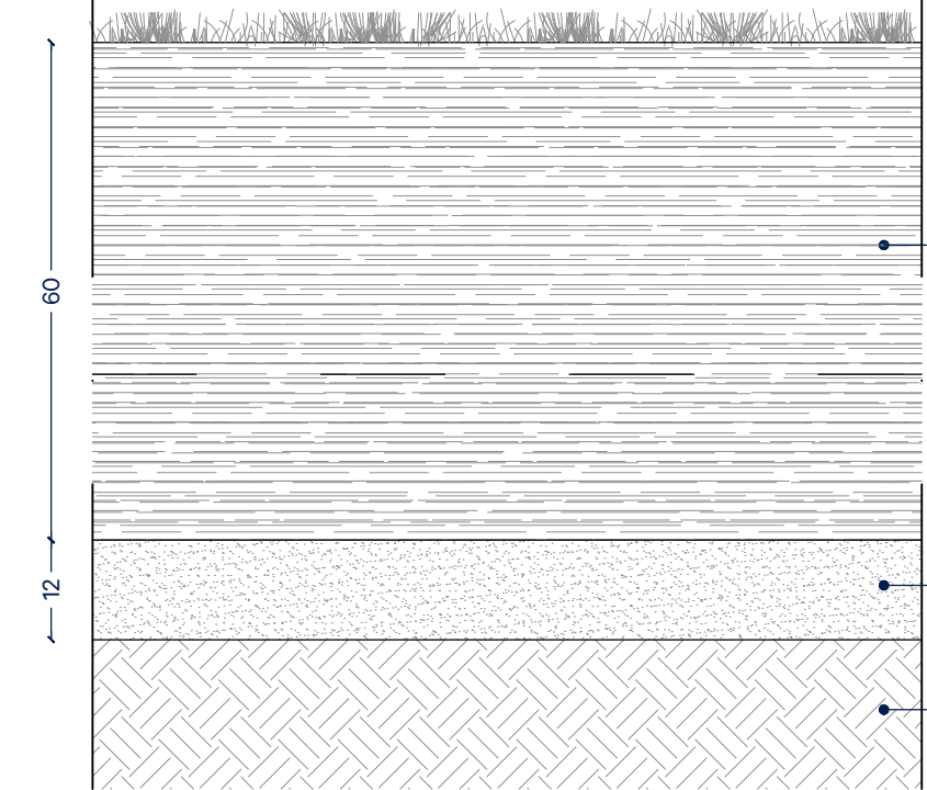
C02 - Aiuole scala 1:10
