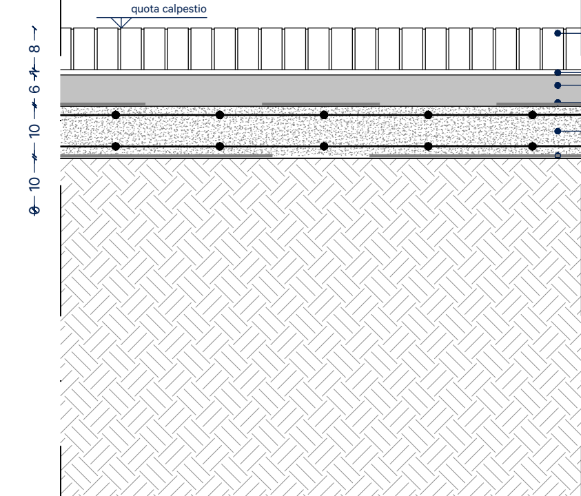
C03 - Pavimentazione in cubetti di porfido scala 1:10
