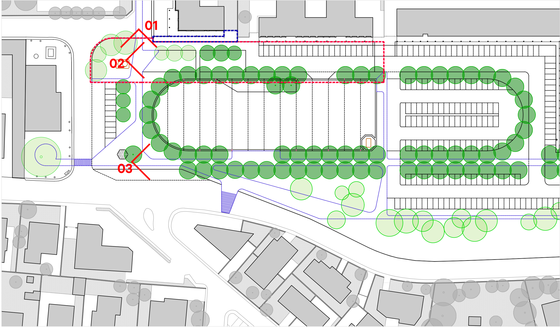
PLANIMETRIA GENERALE sc. 1_500
