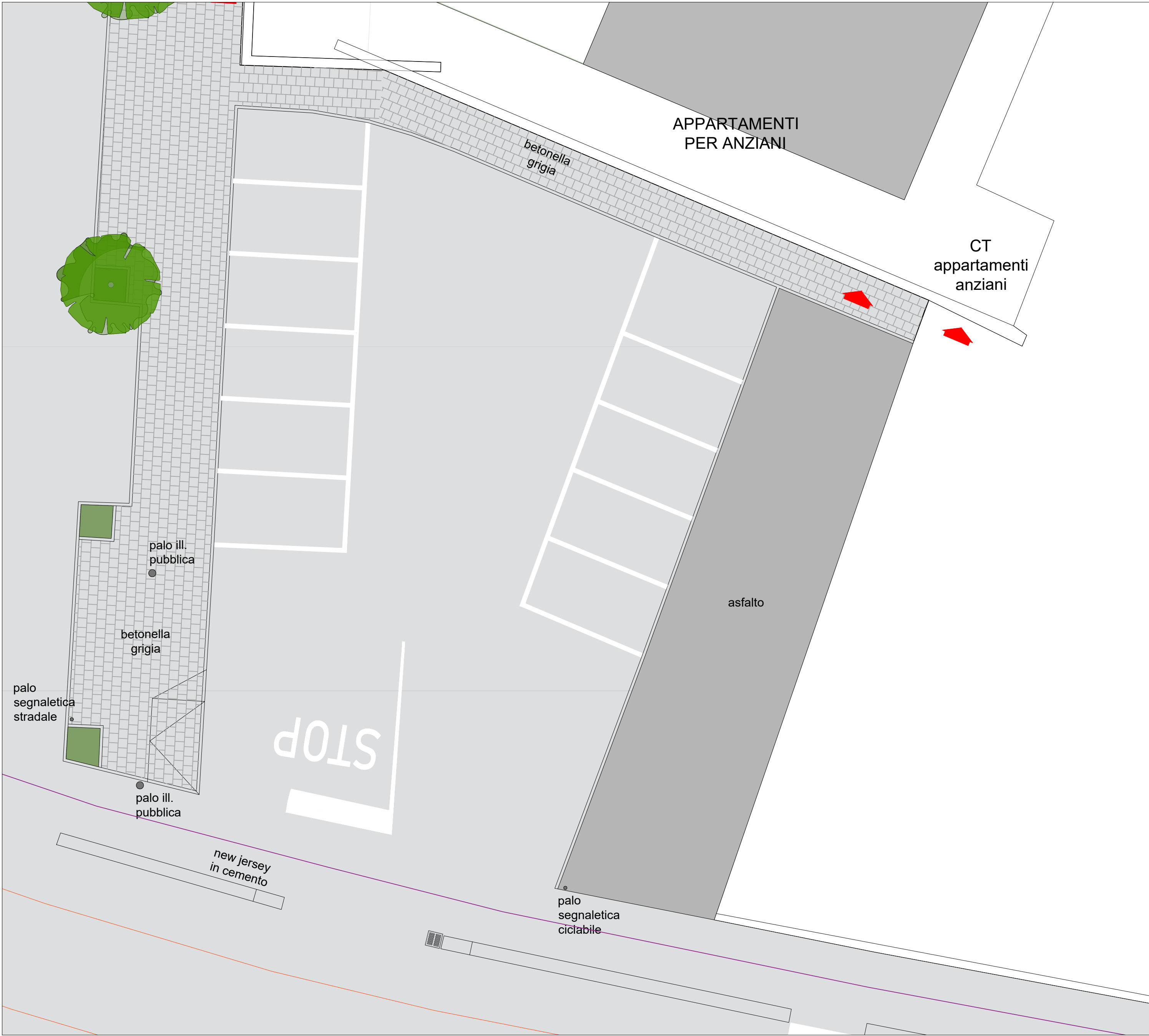
PLANIMETRIA PARCHEGGIO DA MODIFICARE - STATO DI FATTO scala 1:100
