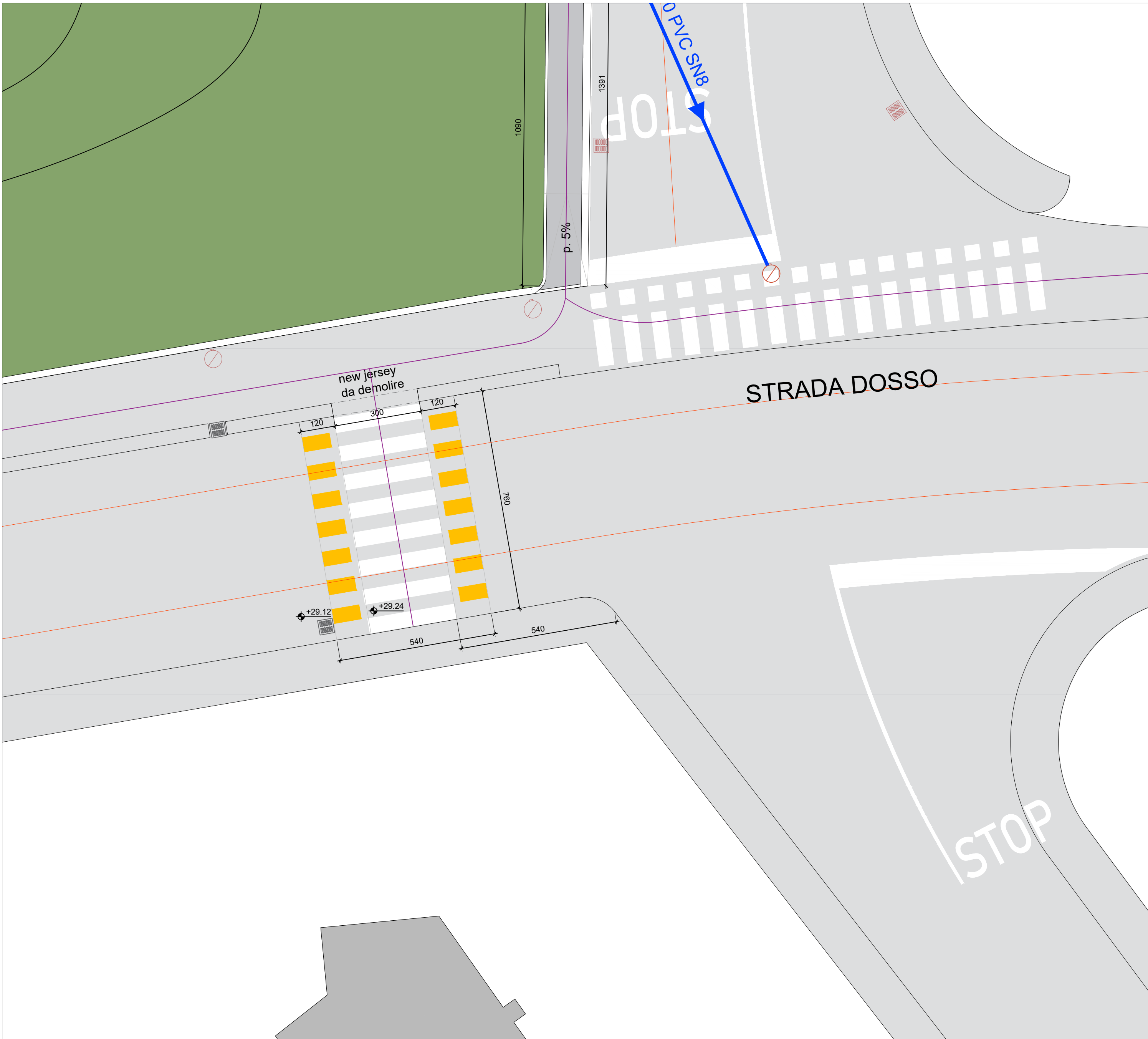
PLANIMETRIA ATTRAVERSAMENTO RIALZATO - STATO DI PROGETTO scala 1:100
