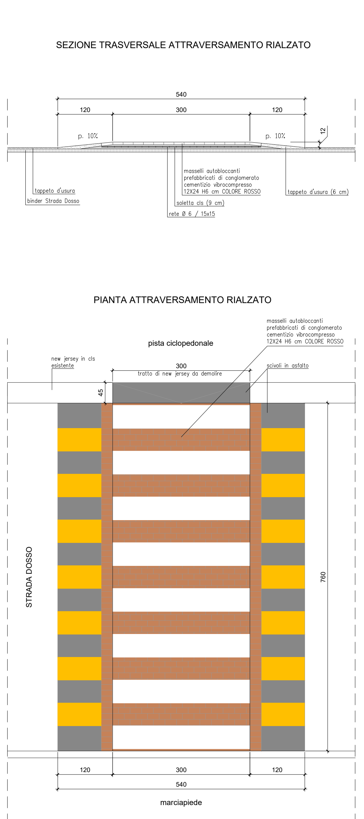
PARTICOLARE ATTRAVERSAMENTO RIALZATO scala 1:50
